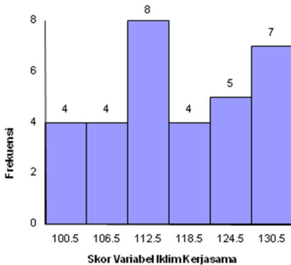
Gambar 2. Histogram Distribusi Skor Variabel Iklim Kerjasama
